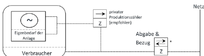
Messanordnung B2: Überschussmessung bei Kleinanlagen
